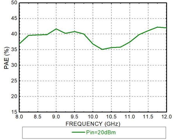
PAE
