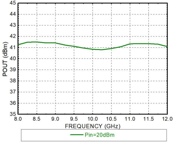
输出功率
